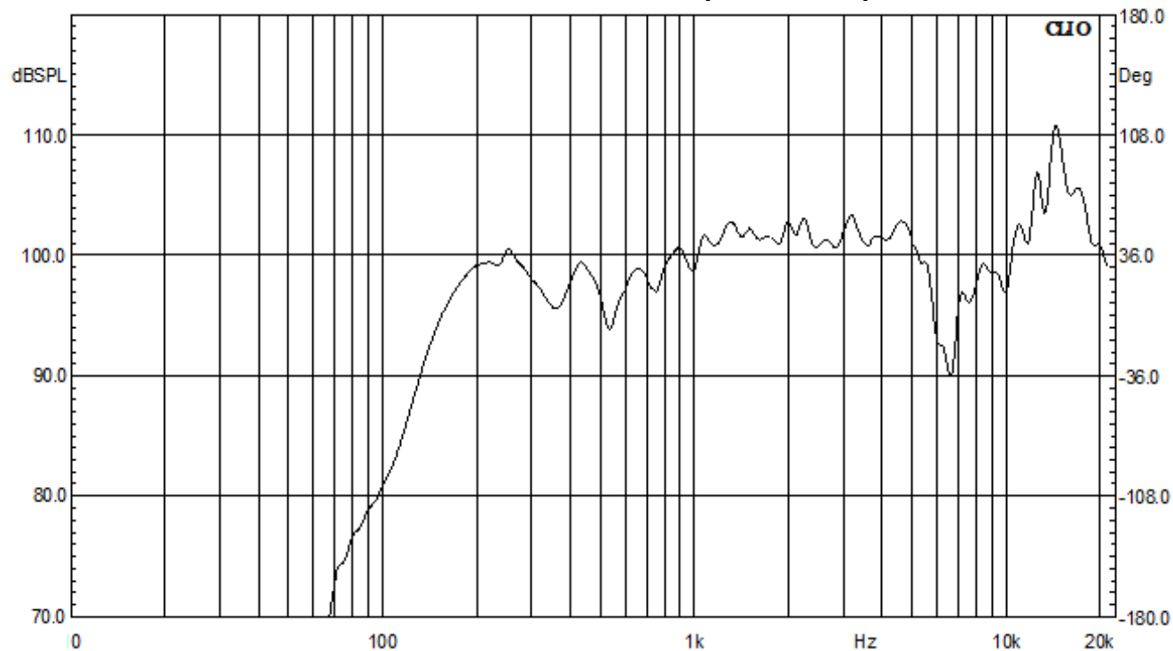
АЧХ RPA-8, 15Вт
